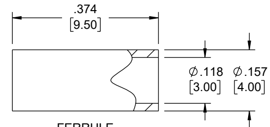
FERRULE
