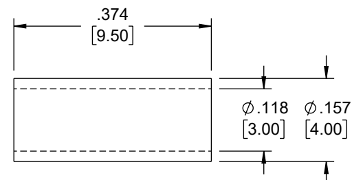
FERRULE
