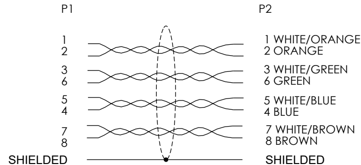
WIRING MAP
